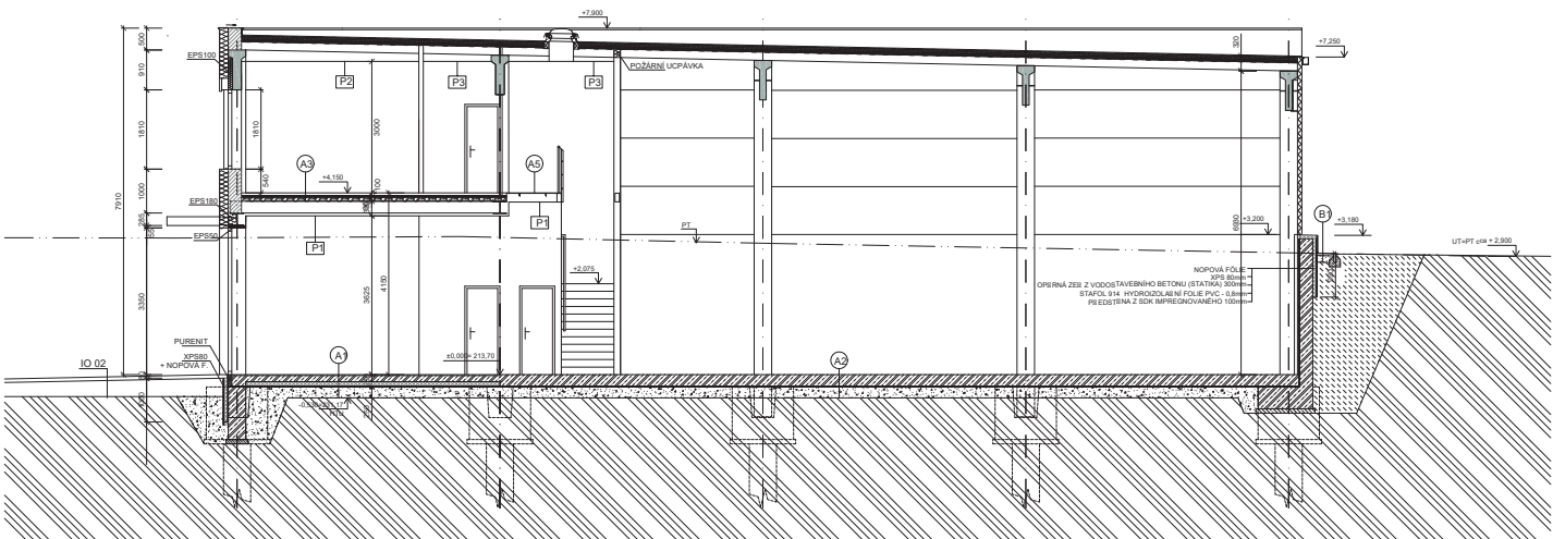
ŘEZ B-B'
