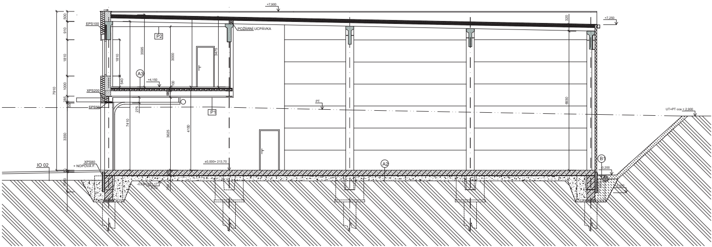
ŘEZ A-A'
