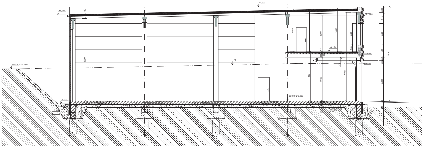
ŘEZ A-A'
