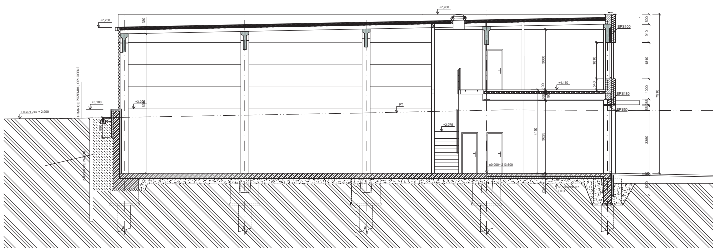
ŘEZ B-B'
