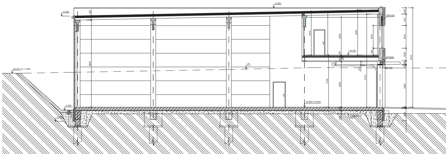
ŘEZ A-A'
